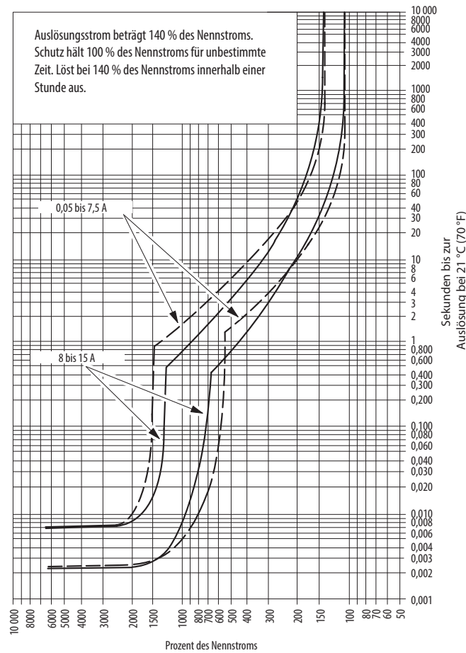
Zeit-Strom-Kurve – 1492-GH
